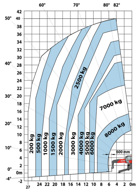
Machine sur stabilisateurs abaissés avec fourches
