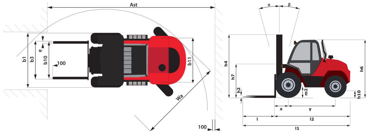
M 40-4 D ST5 - Schémas d'encombrement
