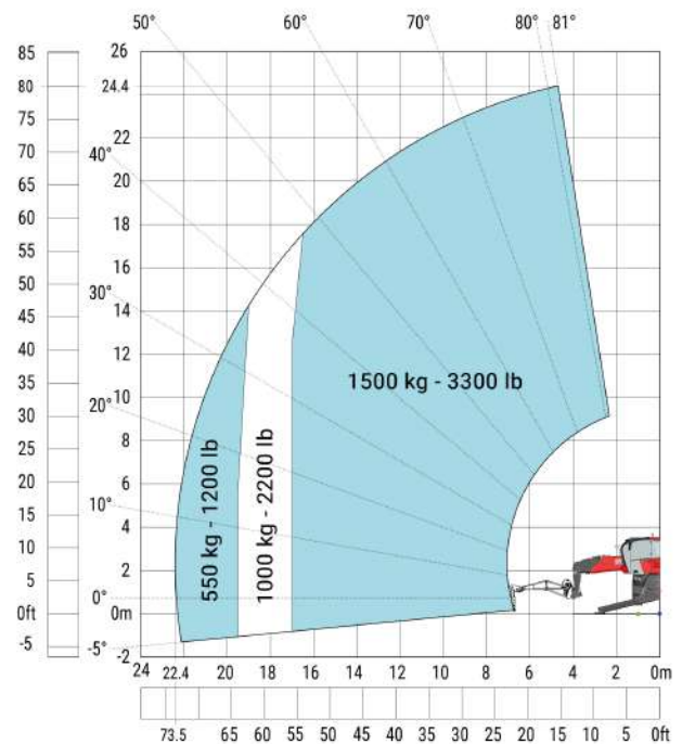
Machine sur stabilisateurs abaissés avec potence 1500 kg
