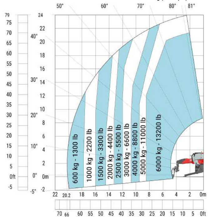
Machine sur stabilisateurs abaissés avec treuil 6000 kg (Métrique)
