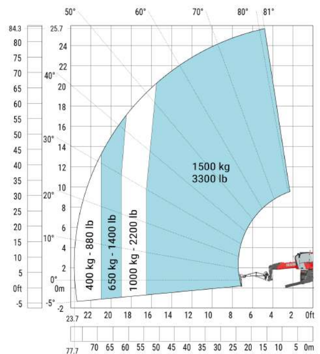
Machine sur stabilisateurs abaissés avec potence 1500 kg
