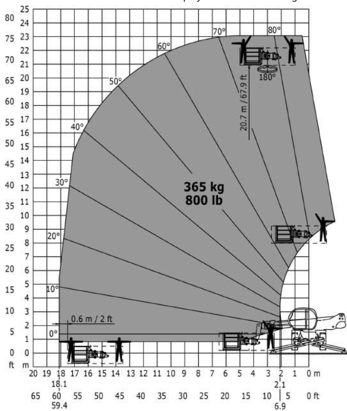
Rotation sur stabilisateurs déployés avec nacelle 365 kg
