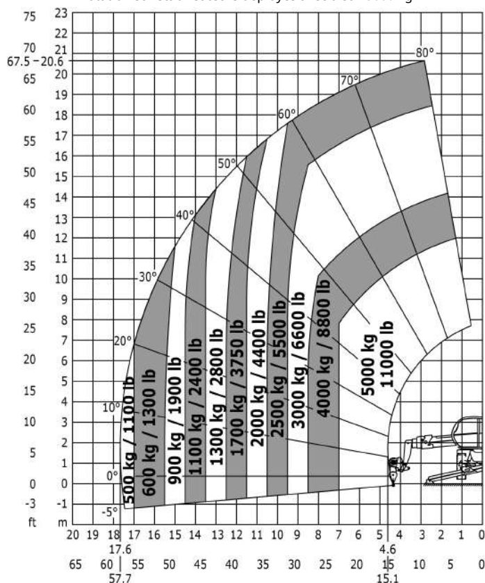
Rotation sur stabilisateurs déployés avec treuil 5000 kg
