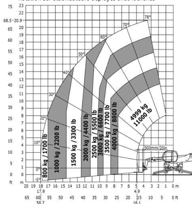
Rotation sur stabilisateurs déployés avec fourches
