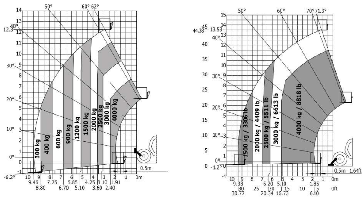
Machine sur pneus avec fourches - avec correcteur de d v rs
