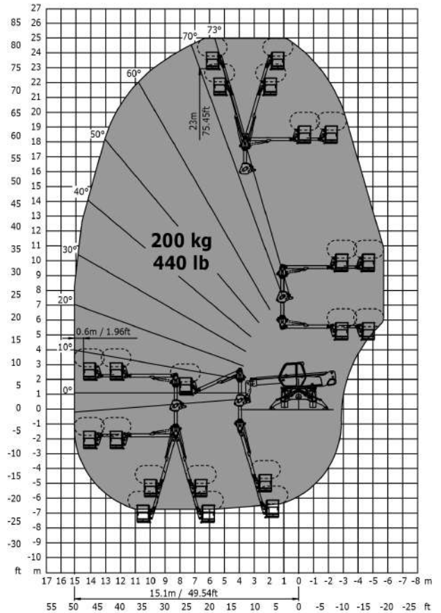
Rotation sur stabilisateurs déployés avec 3D positif / négatif
