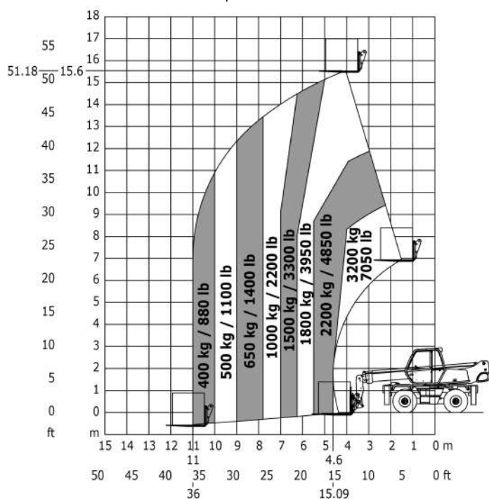
Machine sur pneus avec fourches
