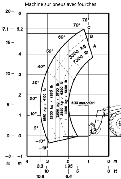
Graphique de charge conforme à la norme EN 474-3 (80%)
